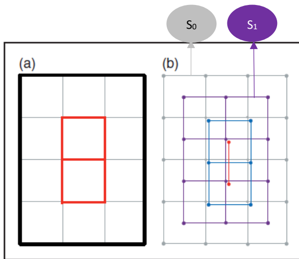
شکل ۹. گراف درخت
