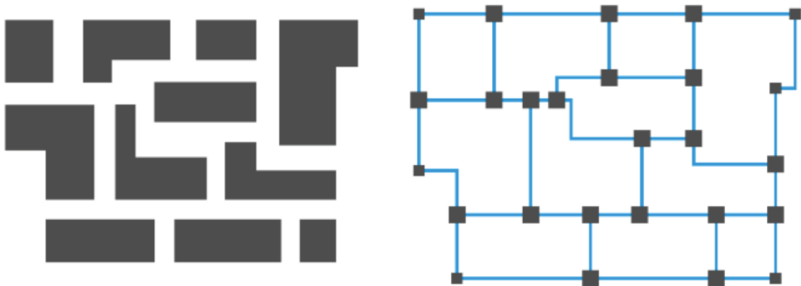
شکل ۴. گراف اولیه
