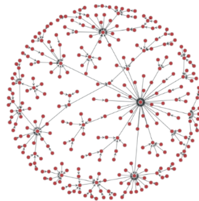
شکل ۸. گراف دوگان
