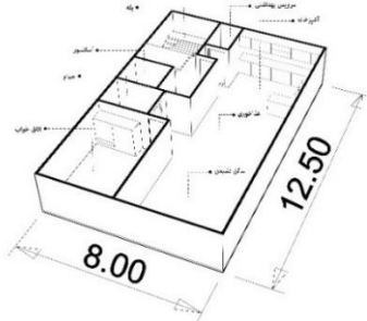
شکل ۴. نمونه‌ی کوچک‌ترین بلوک با در نظر گرفتن مشاعات طبق مقررات ملی ساختمان
