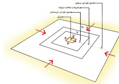
شکل ۵. دیاگرام محاسبه‌ی ابعاد بزرگ‌ترین بلوک
